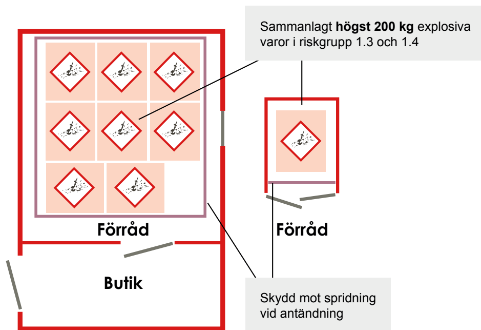
Bild 44: Skiss över förvaringslösning enligt alternativ 2.
