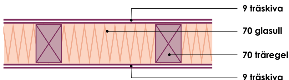
Bild 35: Exempel på EI30-avskiljning med träskivor på träreglar och glasull (mått i mm).
